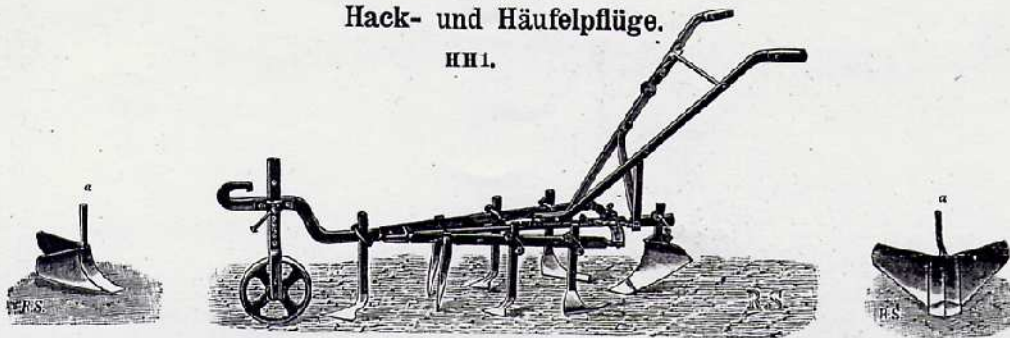
155. Hack- und Häufelplug, Marke HH1, stellbar für Reihenweite von 33—55 cm. Gewicht 33 kg. Zum Reinigen und Lockern der Reihenzwischenräume in Kartoffeln, Rüben u. s. w. Preis M. 33.—. Der Anhilfler kann auf Wunsch mit stellbaren Streichblechen (a) unter entsprechender Mehrberechnung geliefert werden. Preis M. 37.—.
