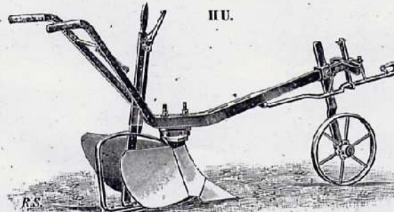
158. Häufelplug, Marke HU, mit stellbaren Streichblechen und Einstellung derselben von den Handhaben aus. Dargestellt mit Gründel vom Weinbergspfluge WB, Abb. 119, mit festen Handhaben. Gewicht 41 kg. Preis M. 30.—. Kann auch mit Gründel vom Universalpfluge D7 mit festen Handhaben geliefert werden.
